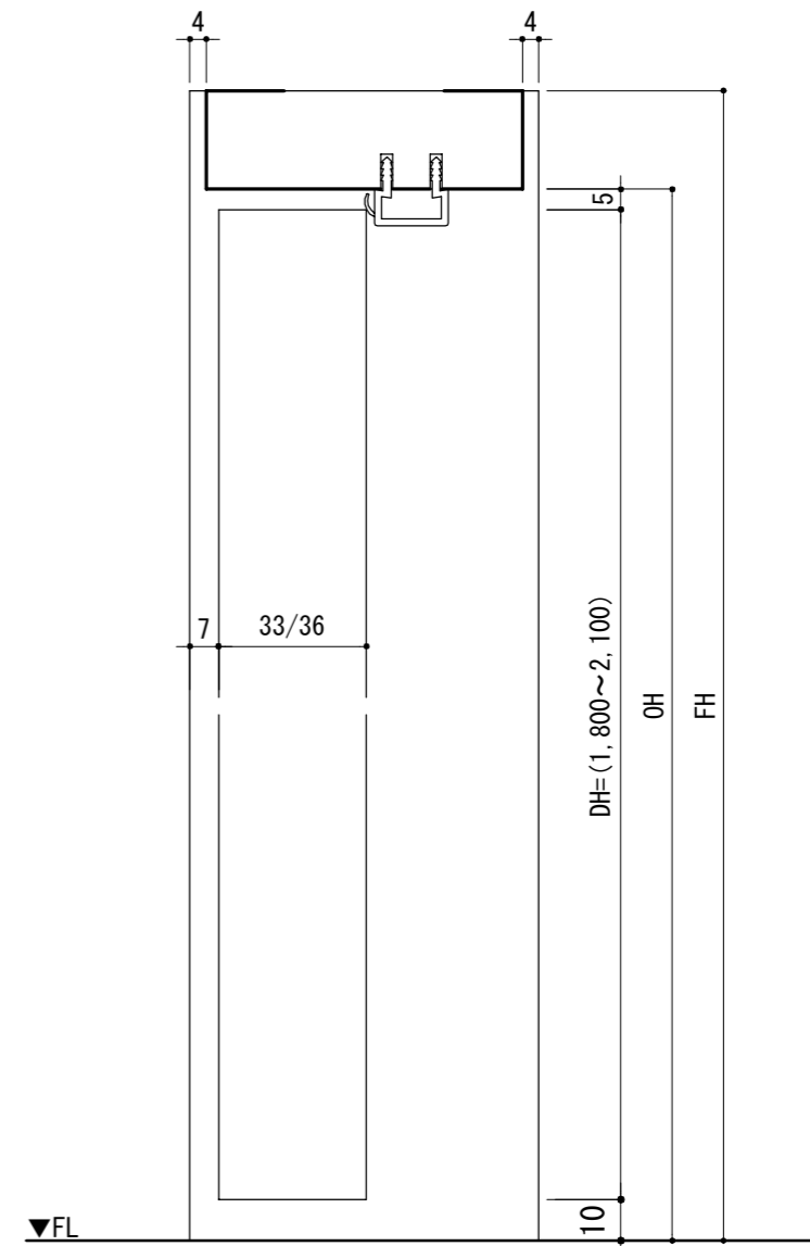
縦断面図 1/2
