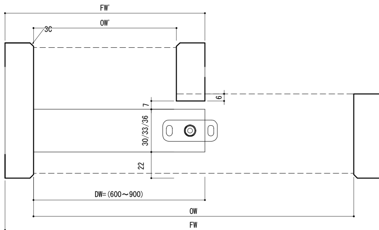
横断面図 1/2
