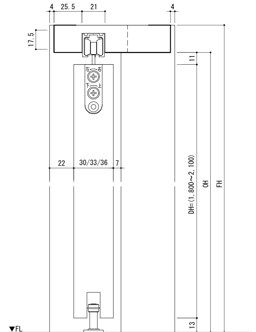
縦断面図 1/2
