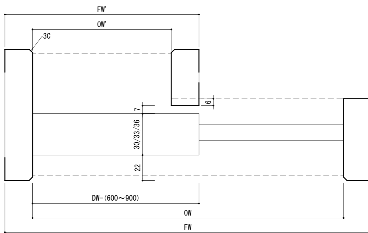
横断面図 1/2
