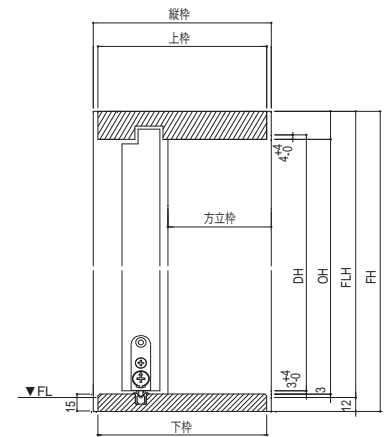
縦断面図
